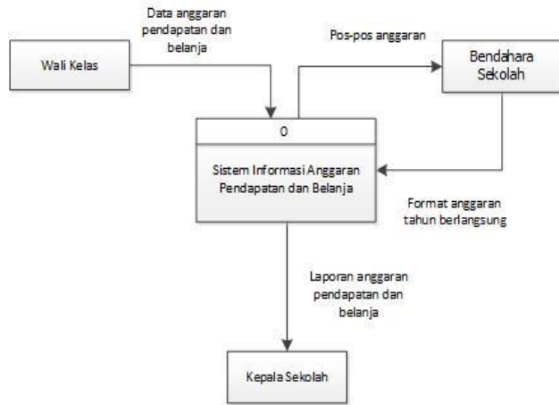
Gambar 3.1 Diagram Konteks Yang Diusulkan
