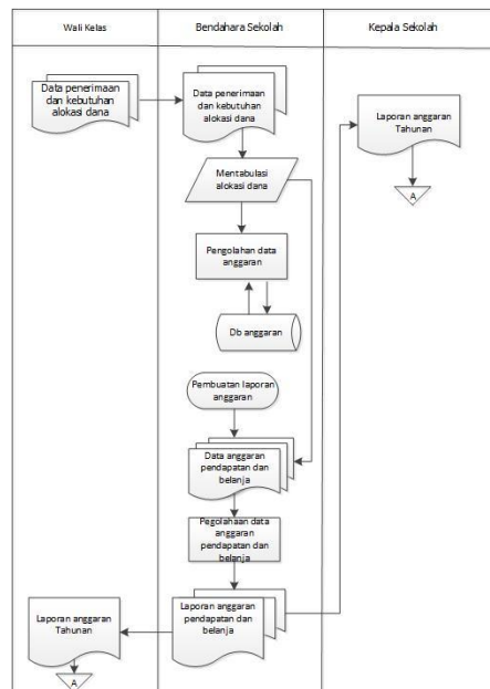
Gambar 3.4 Sistem Informasi Yang Diusulkan
