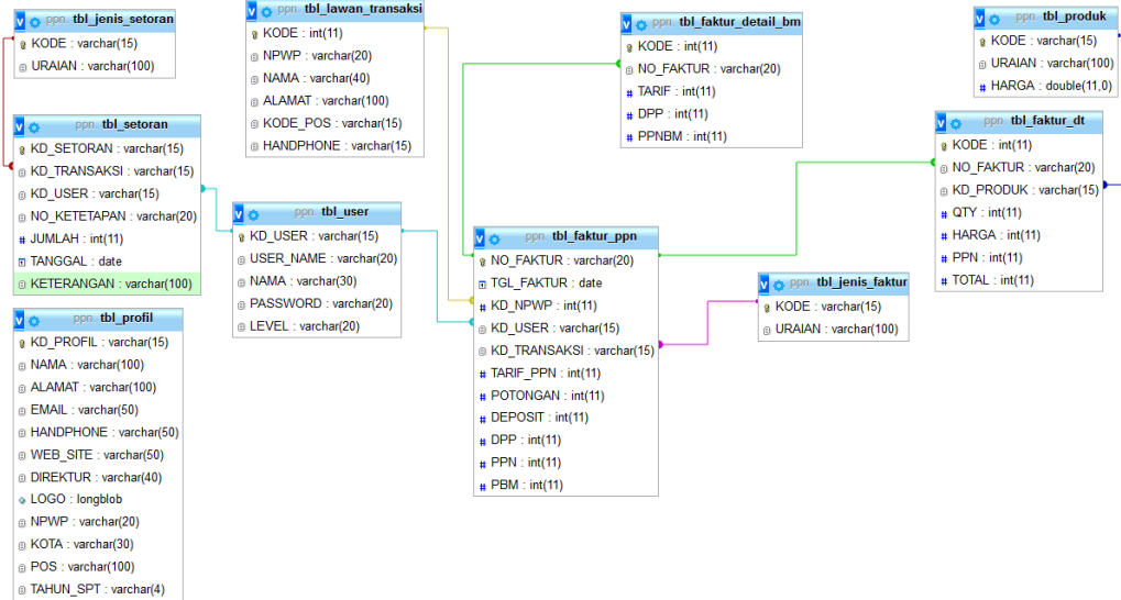
Gambar 3. Relasi Database
