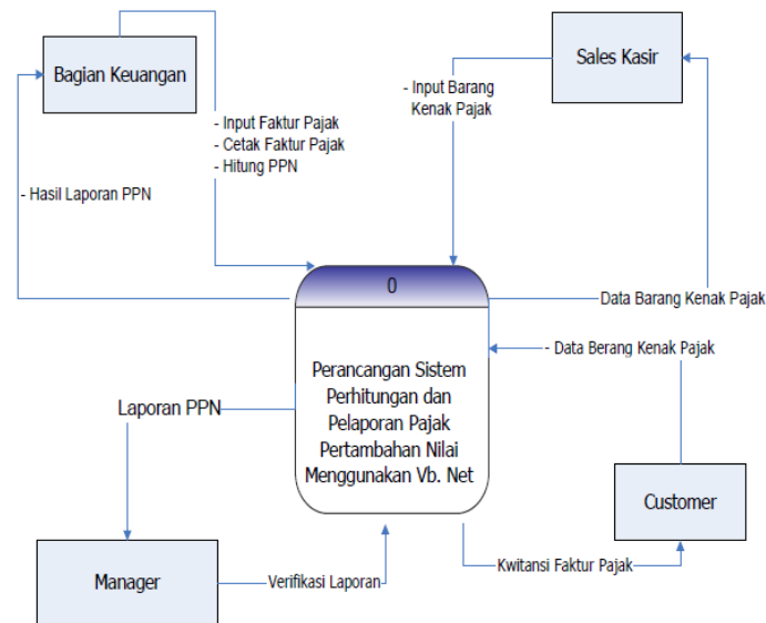
Gambar 1. Diagram Konteks
